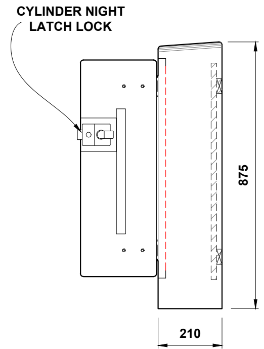
Elevation (D) (r/h side) Door Open
